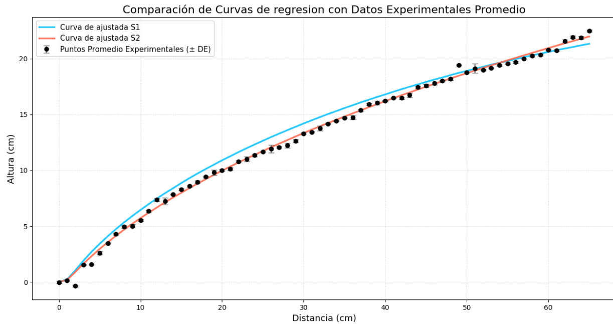
Figure 5: Comparación de las curvas de regresión obtenidas a partir de los datos de la Sesión 1 (Regresión S1, línea azul) y la Sesión 2 (Regresión S2, línea coral) con los puntos experimentales promedio de la Sesión 2 (puntos negros con barras de error de desviación estándar). Los datos experimentales corresponden a la altura de deformación ( y ) en función de la distancia radial ( x ) de la lámina elástica.
