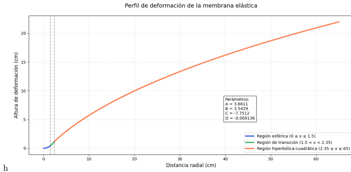
Figure 6: Gráfica de la curva teórica deducida
