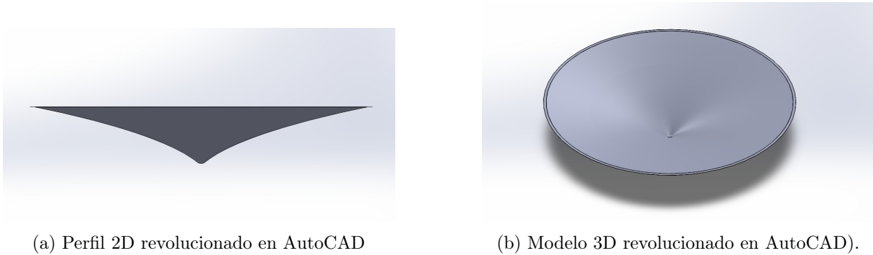
Figure 7: Diseño conceptual del análogo físico tridimensional, derivado del modelo matemático ajustado a los datos experimentales de la Sesión 2. (a) Vista lateral (proyección 2D) del modelo 3D revolucionado, mostrando el perfil de curvatura original que define la superficie. (b) Perspectiva del modelo 3D completo de la superficie de deformación. Ambas representaciones fueron generadas en AutoCAD a partir de la revolución del perfil 2D base alrededor de su eje central, definiendo la geometría para la simulación de la curvatura de la tela.
